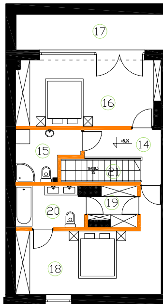
PIĘTRO 2
